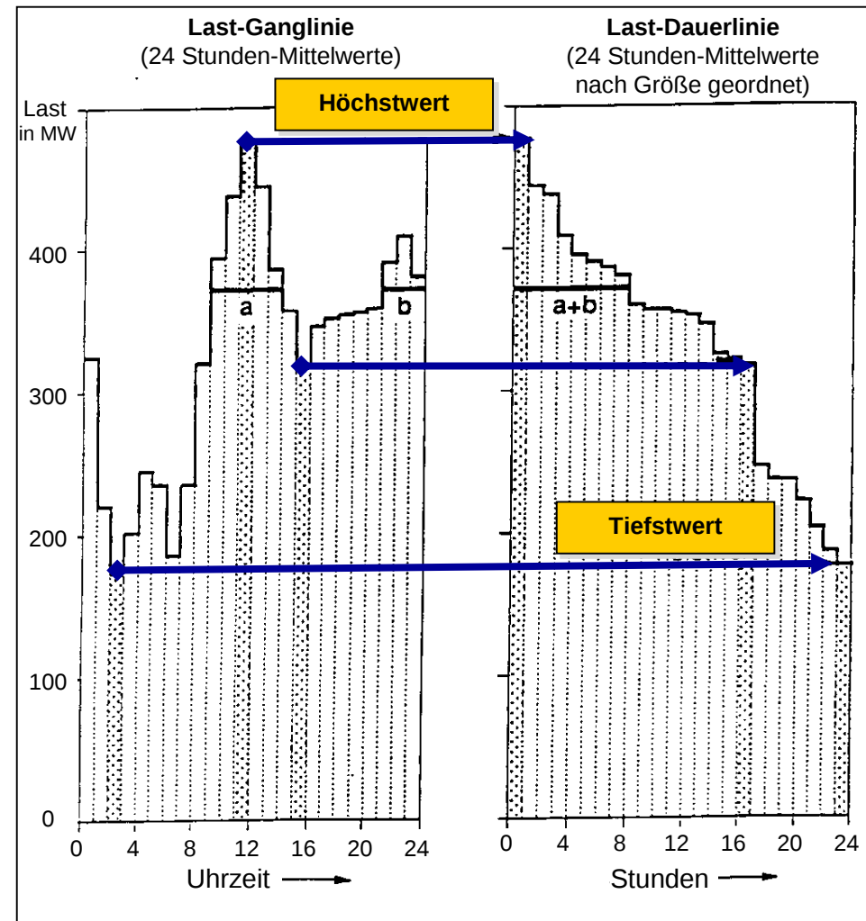
Zusammenhang zwischen Lastgang- und Dauerlinie
